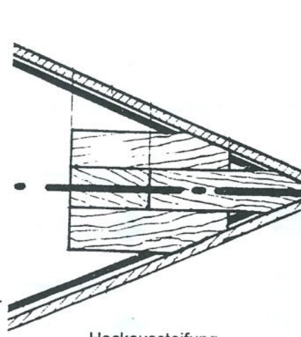
Heckaussteifung
