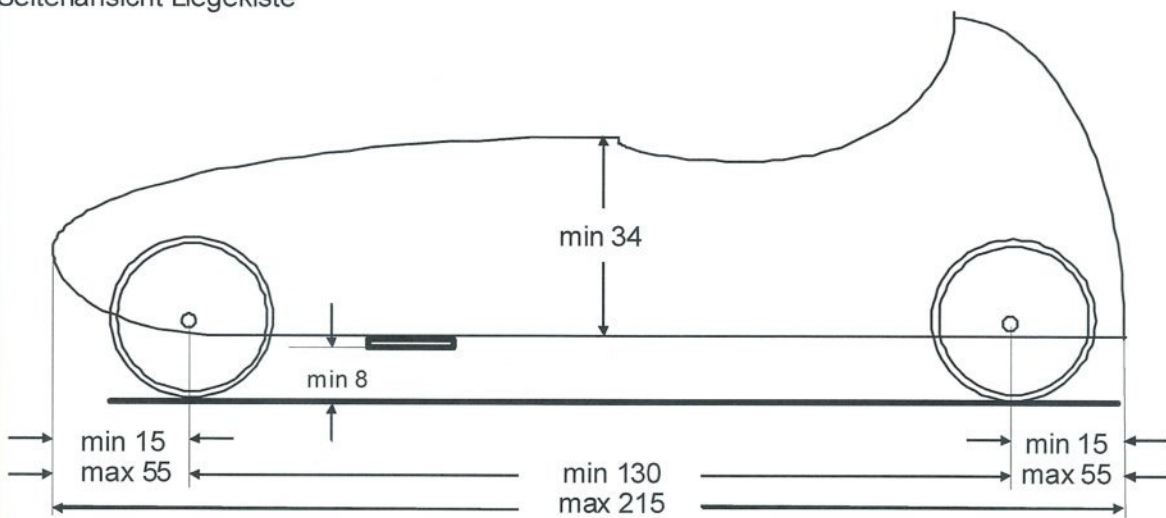
Seitenansicht Liegekiste
