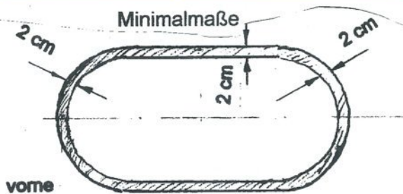
Einstiegsöffnung
