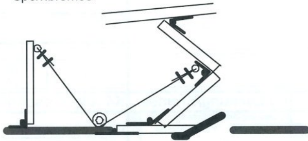
Spornbremse
