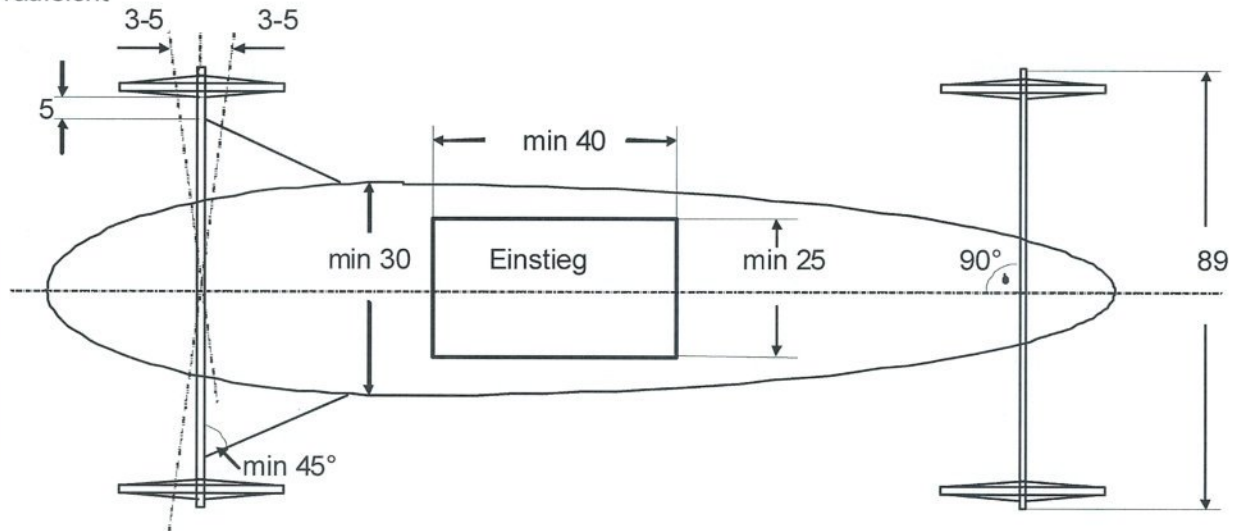
Draufsicht
