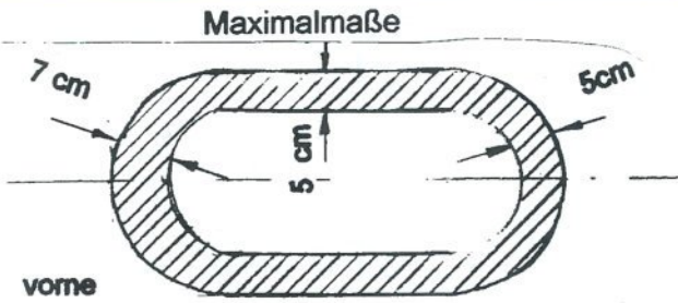
Einstiegsöffnung
