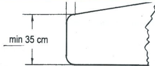
geneigte Deckplatte
